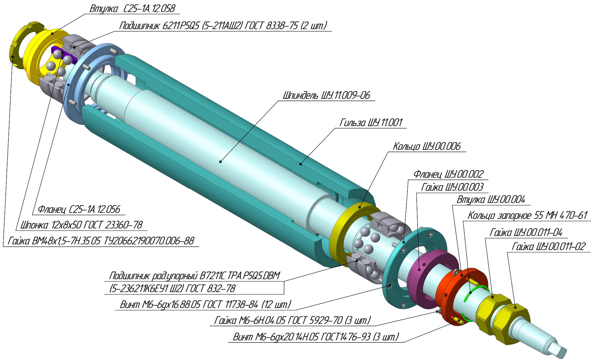
Шпиндель ШУ.11.000-06 СБ (лист 12/12)
