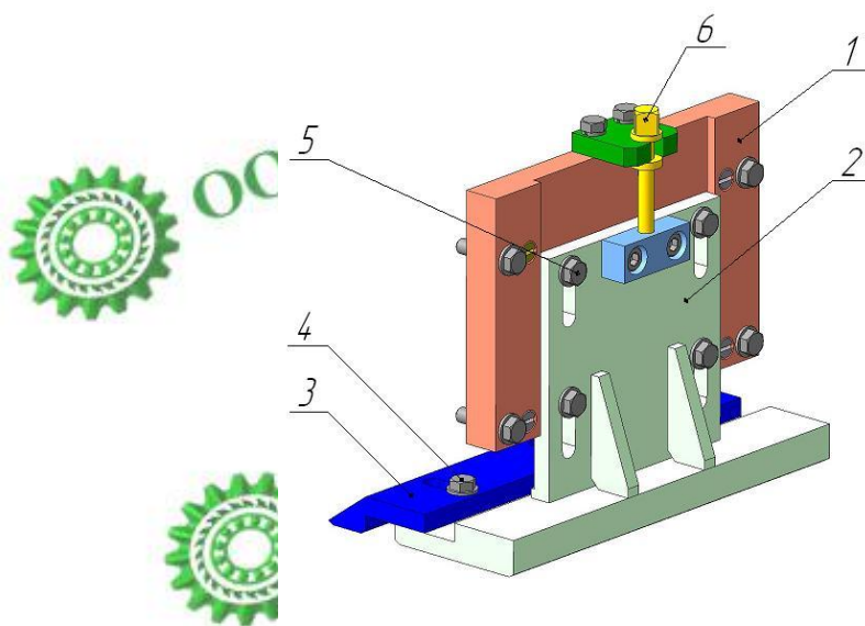
Рис. 21. Прижим задний
