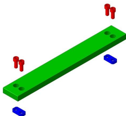
Рис. 4.1. Плита C25-5A.11.100
