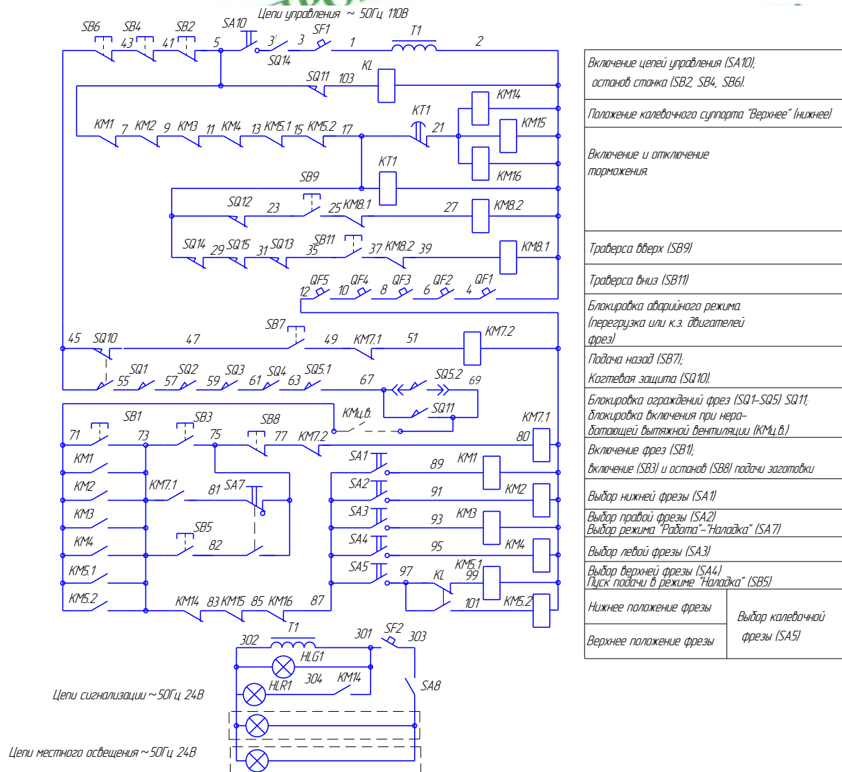
Рис. 23. Схема электрическая принципиальная станка модели C25-5A C25-5A.00.000 Руководство по эксплуатации
