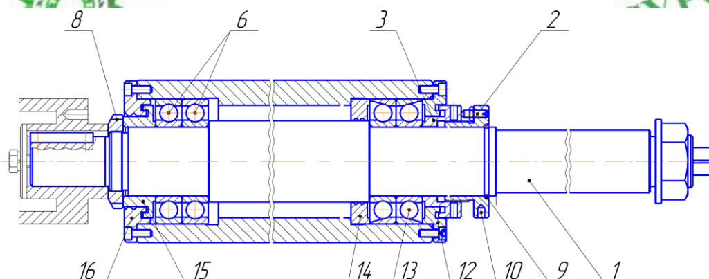
Рис. 32. Шпиндель
