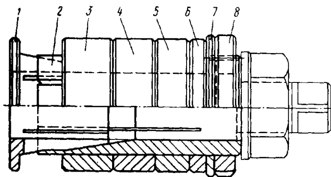
Рис. 4.4. Оправка ИП.01.000
