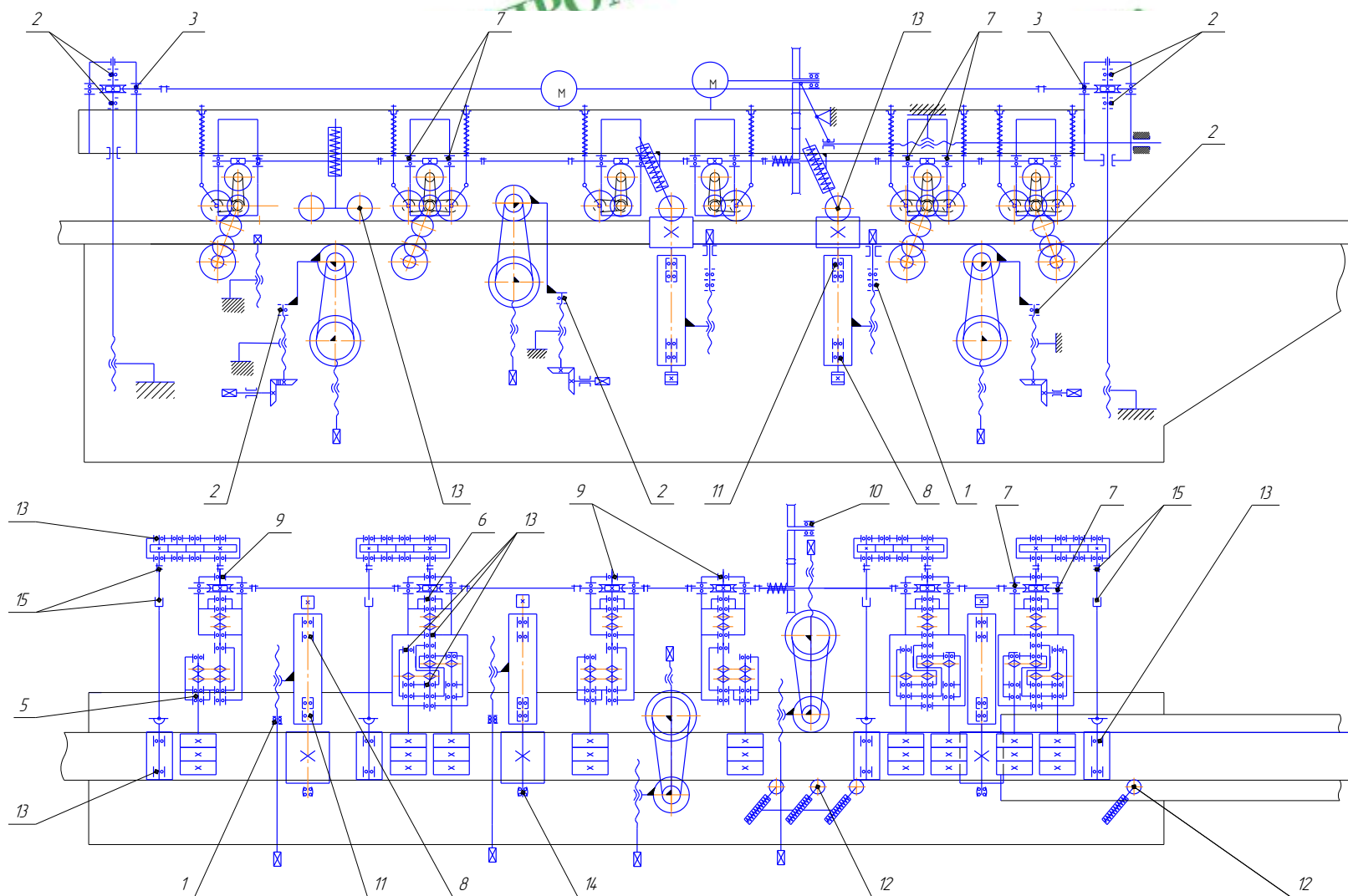
Рис. 36. Схема расположения подшипников
