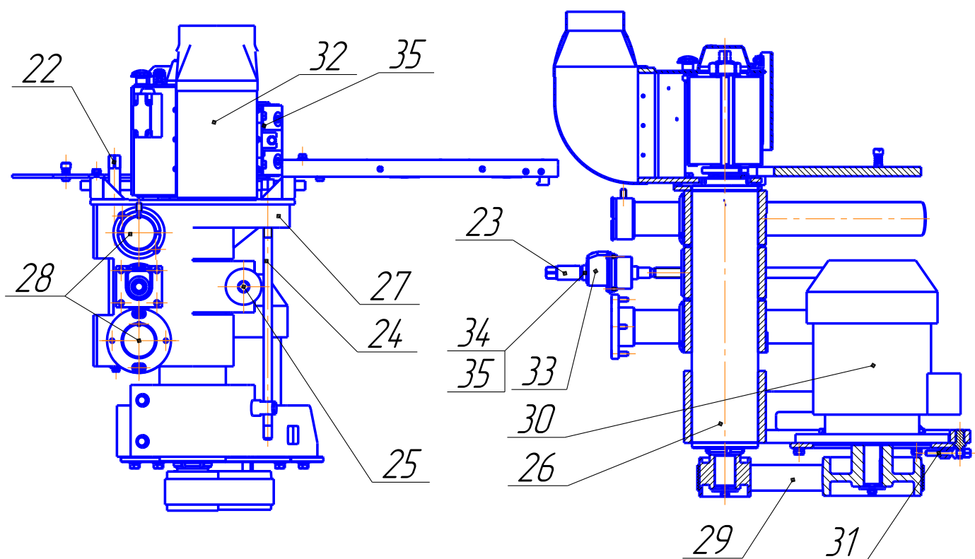
Рис. 16. Суппорт левый
