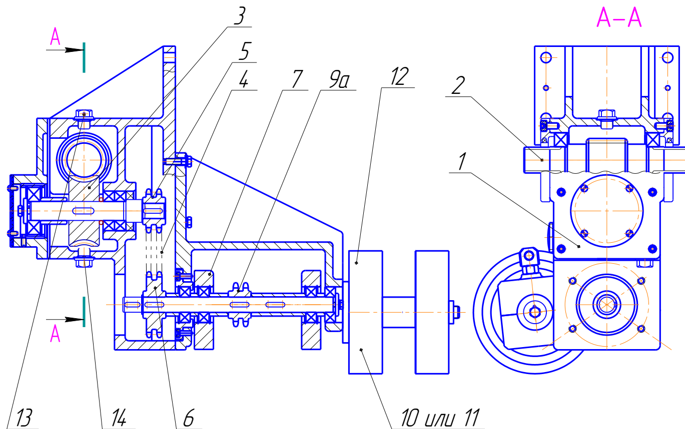
Рис. 12. Модуль привода С16 3.27.000
