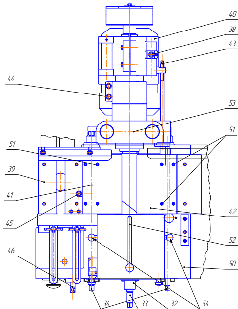
Рис. 18. Суппорт калевочный
