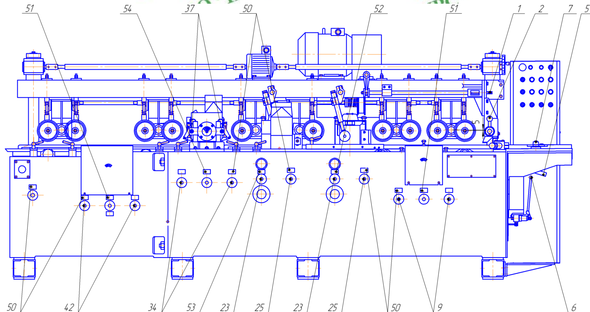
Рис.5 Расположение органов управления станка.
