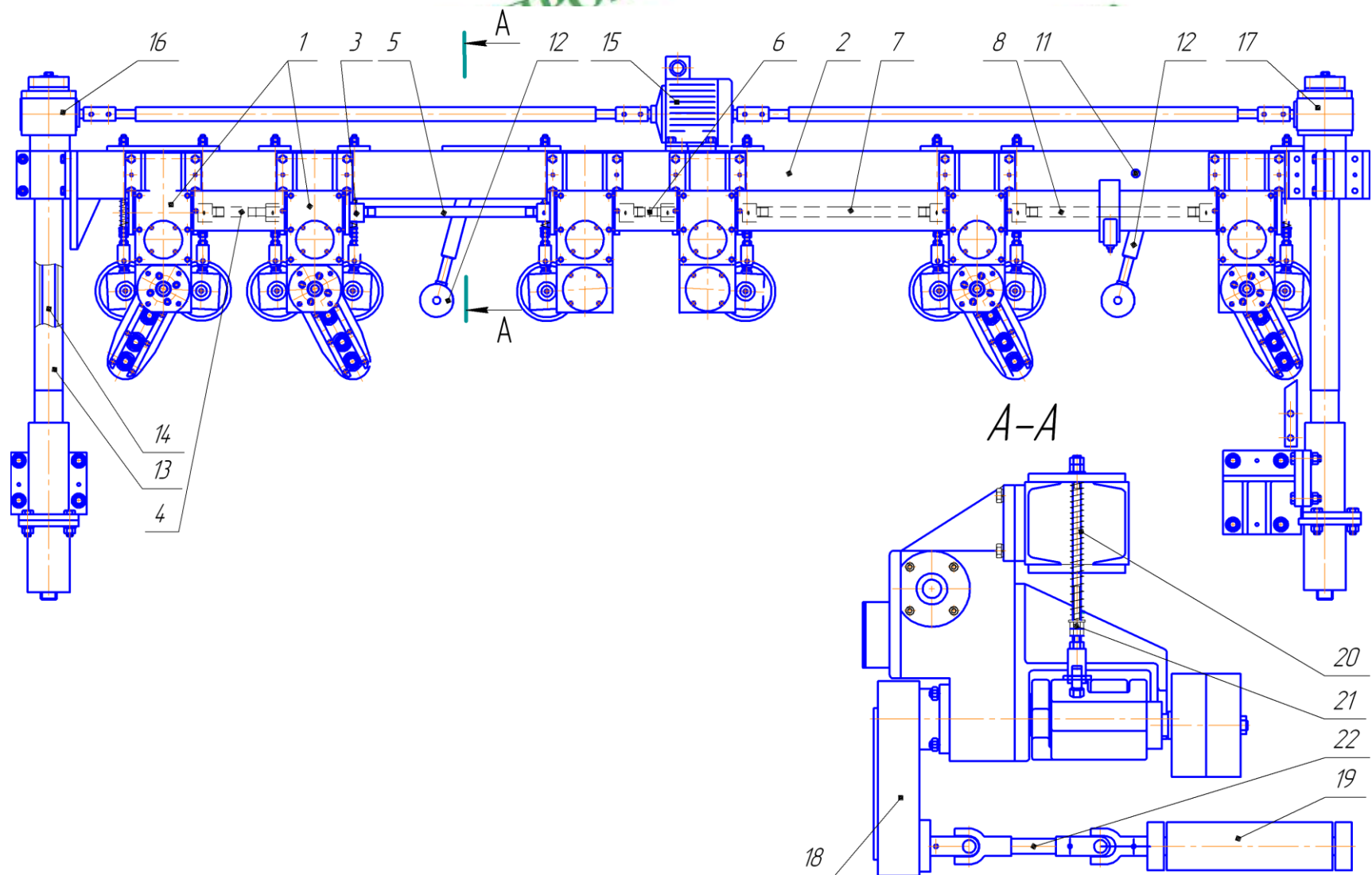
Рис. 10. Механизм подачи
