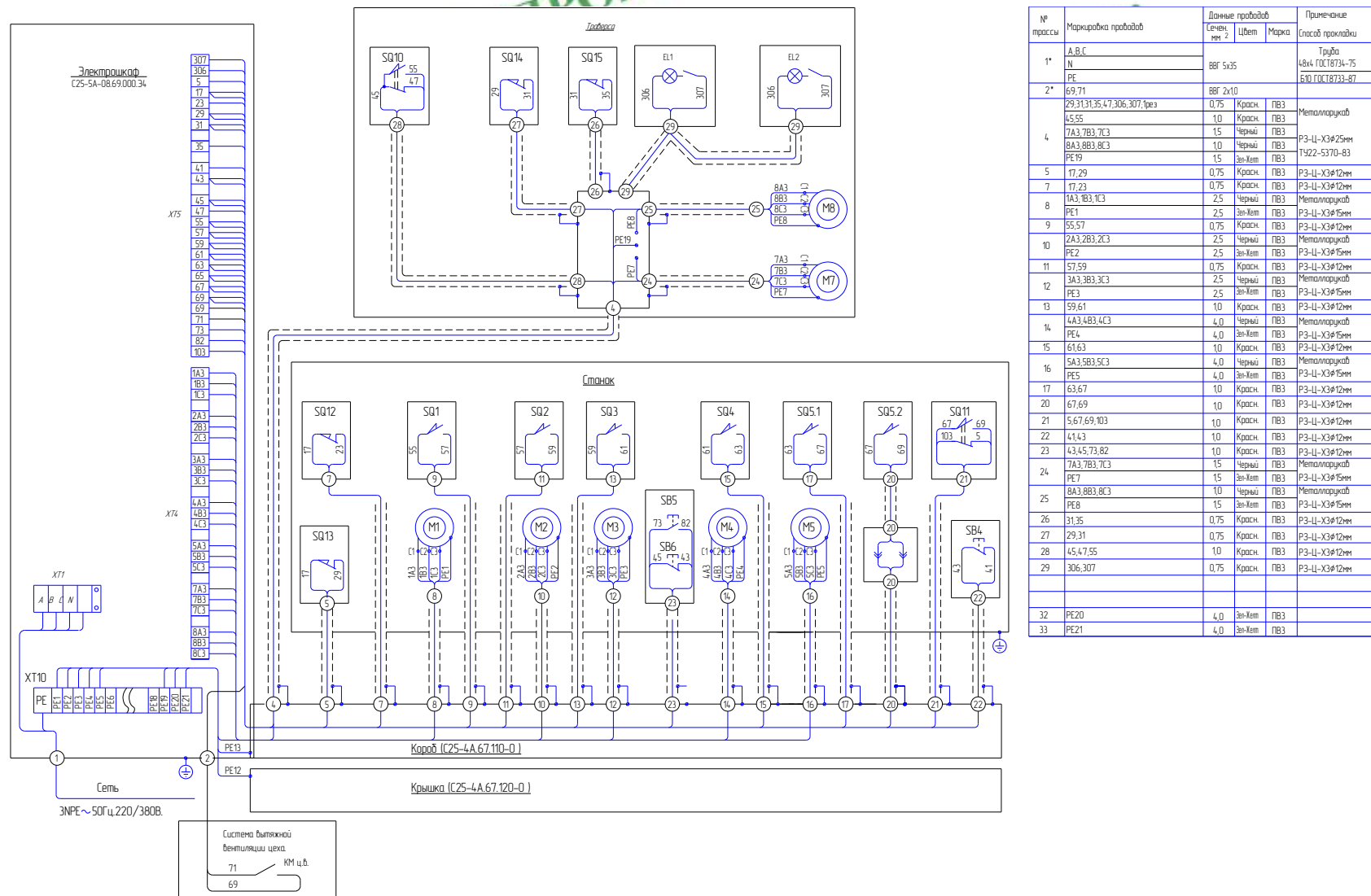
Рис. 24. Схема электрическая общая станка модели C25-5A
