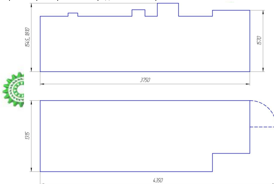
Рис.2 Габаритные размеры
