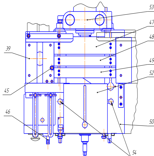
Рис. 19. Суппорт калевочный
