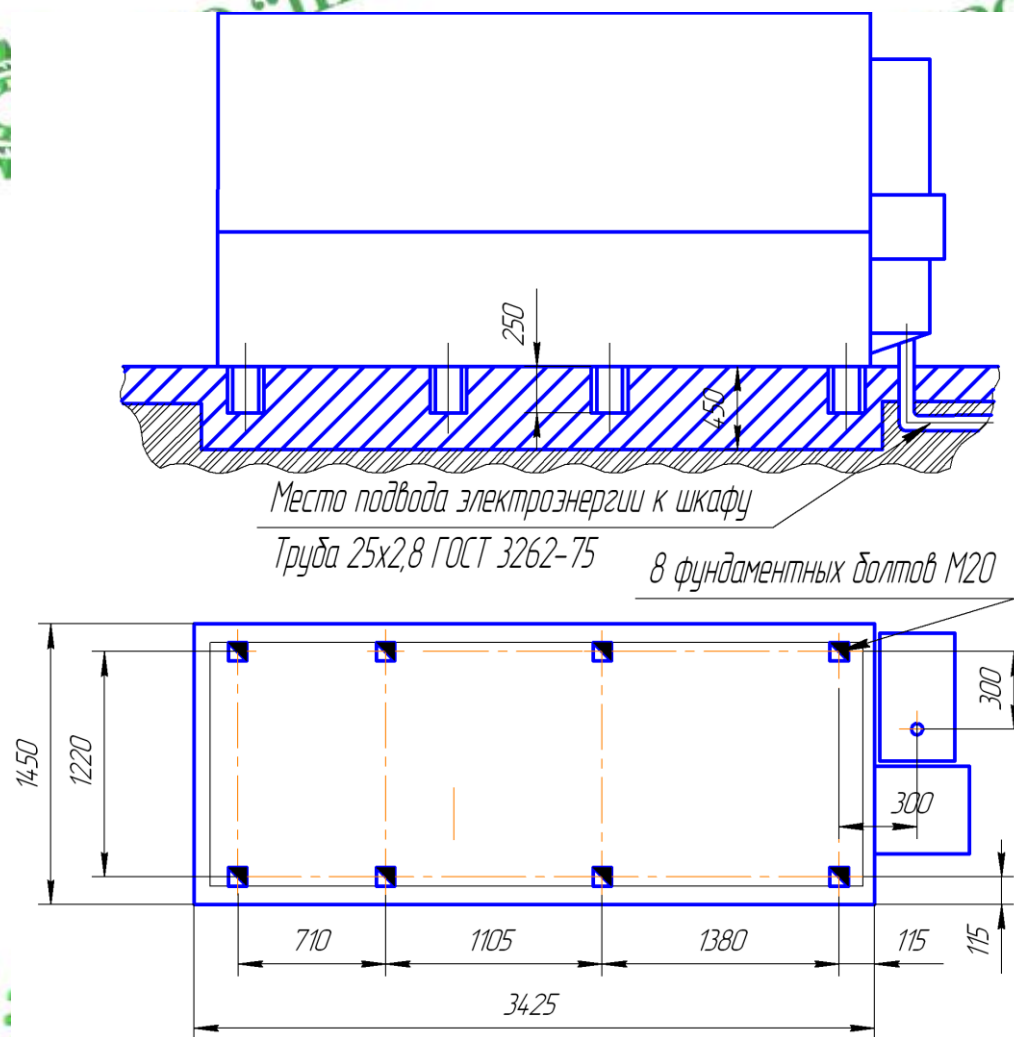
Рис. 29. Схема установки станка
