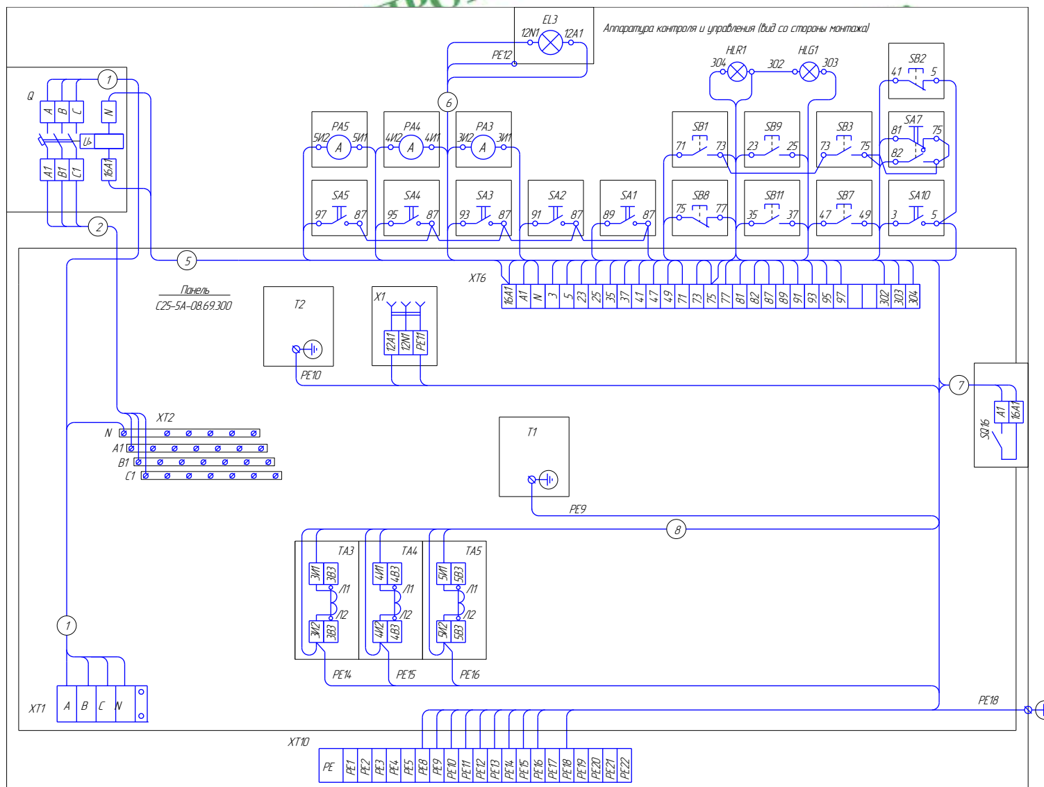
Рис. 25. Схема электрическая соединений станка модели C25-5A C25-5A.00.000 Руководство по эксплуатации
