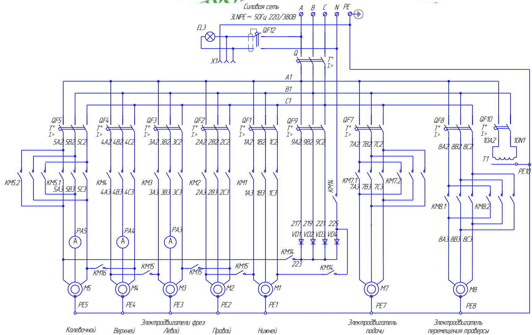
Рис. 22. Схема электрическая принципиальная станка модели C25-5A
