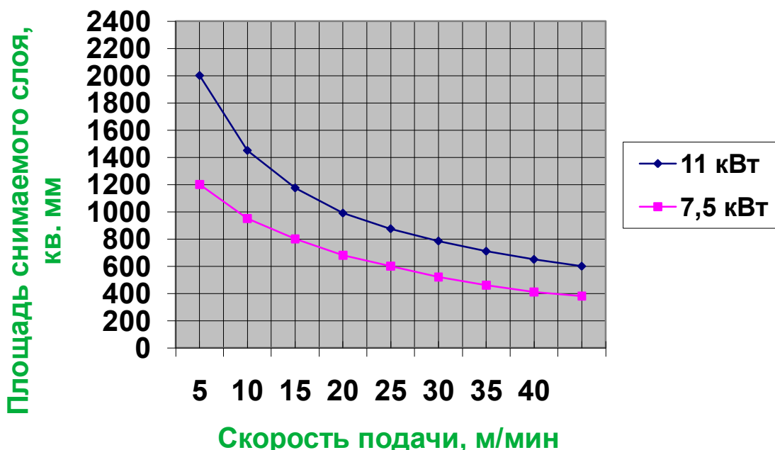
Рис. 29. График зависимости скорости подачи от площади съема
