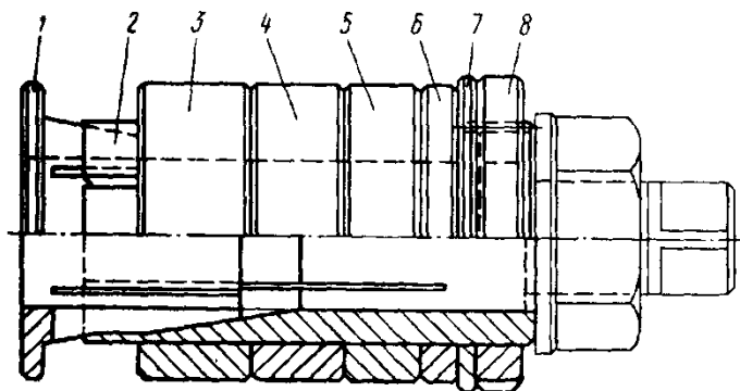
Рис. 4.2. Оправка цанговая правая ИП.07.000
