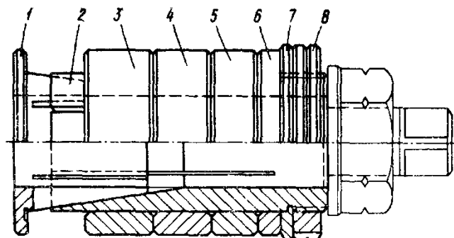
Рис. 4.3. Оправка цанговая левая ИП.08.000
