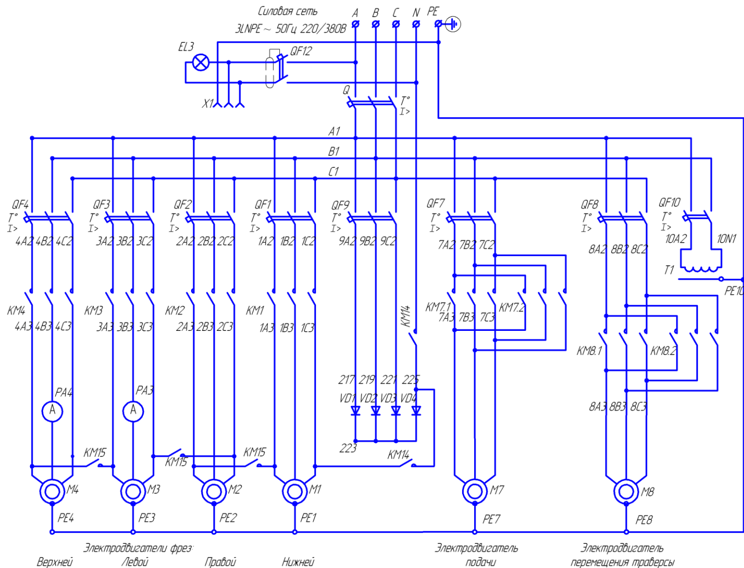
Рис. 18. Схема электрическая принципиальная станка модели C25-4M
