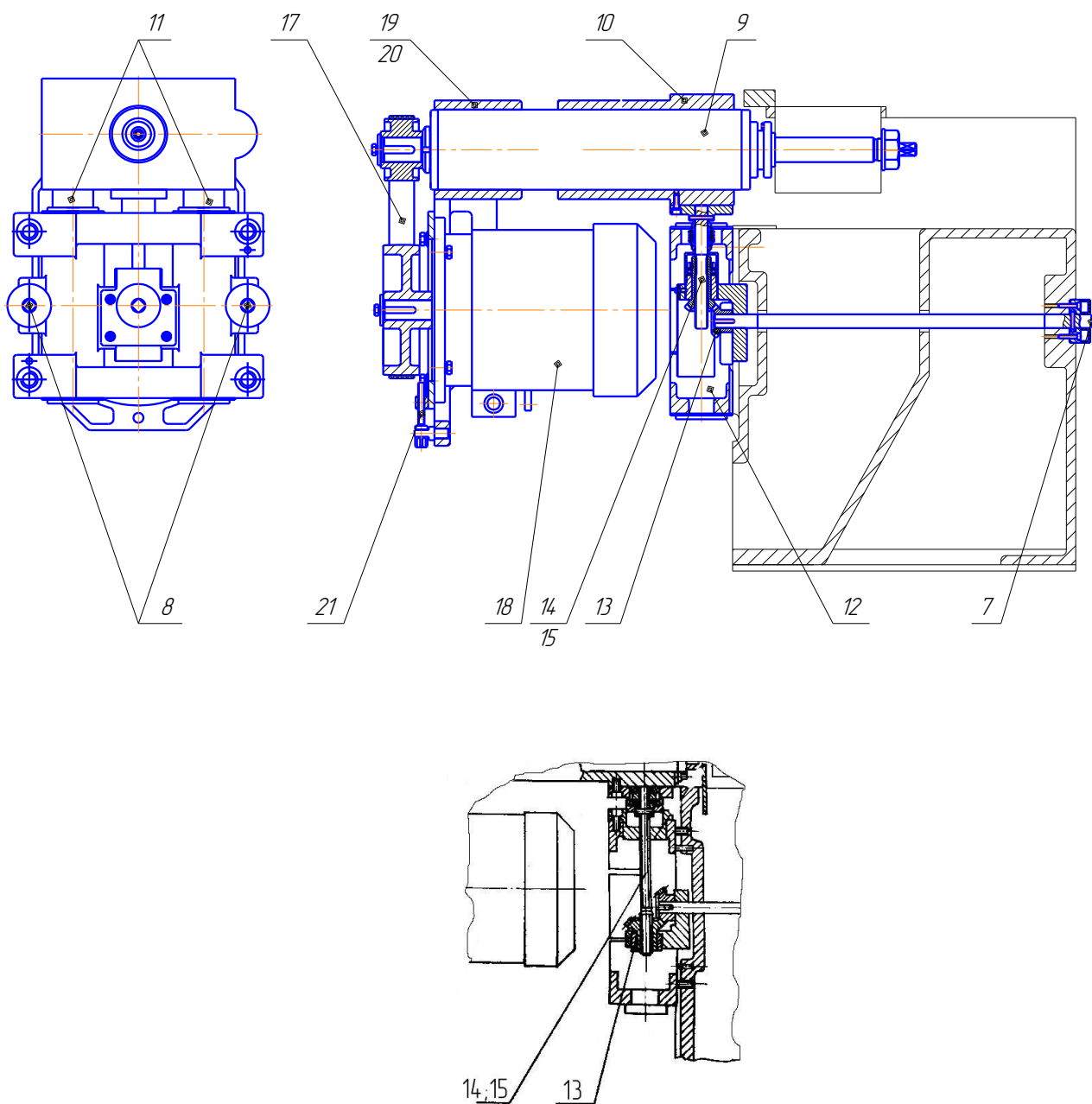
Рис. 12. Суппорт нижний
