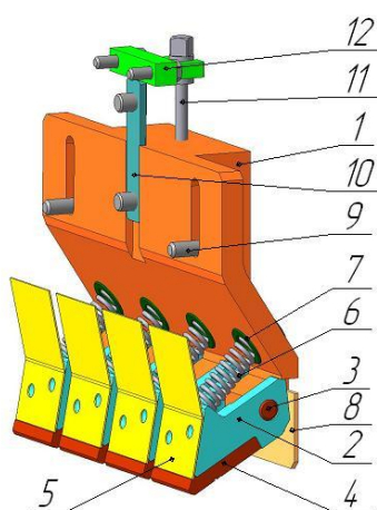
Рис. 16. Прижим передний
