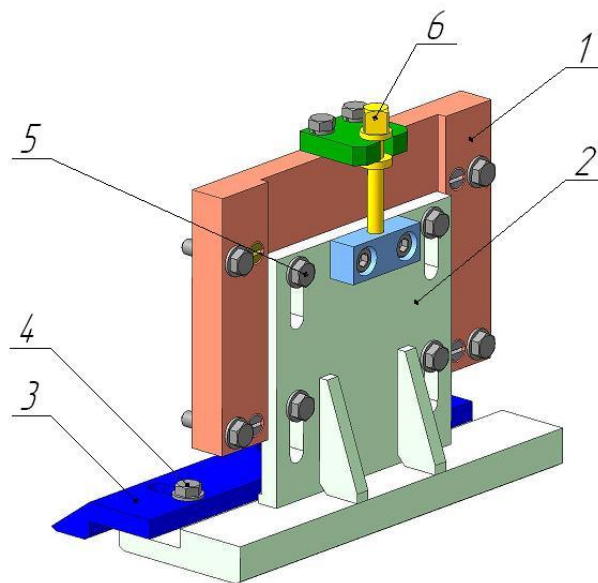
Рис. 17. Прижим задний
