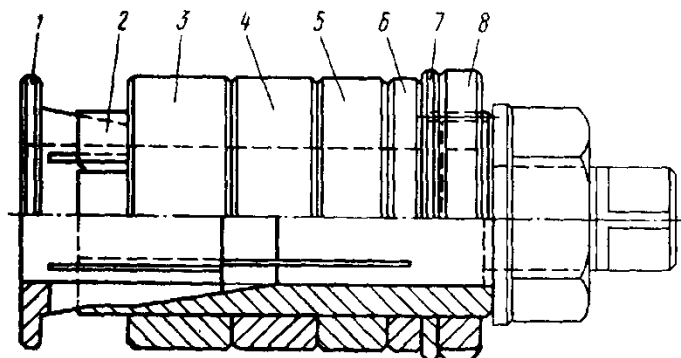
Рис. 4.1. Оправка ИП.01.000
