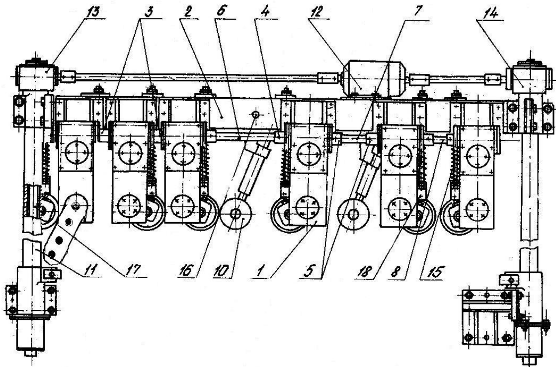
Рис. 8. Механизм подачи
