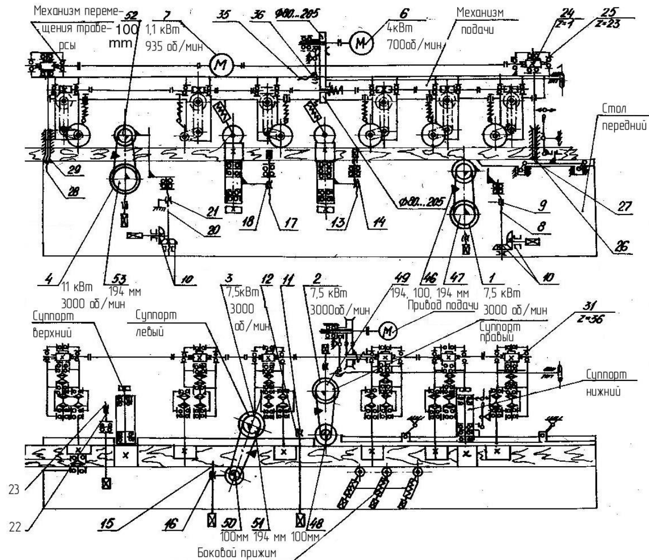
Рис. 6. Схема кинематическая станка С25-4М
