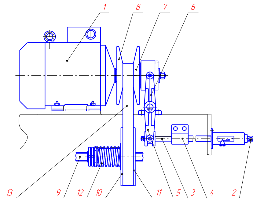
Рис. 7. Привод подачи
