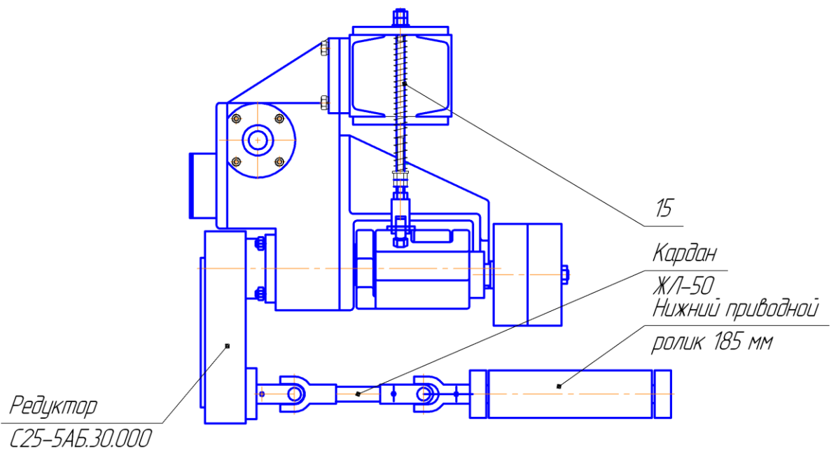
Рис. 9. Механизм подачи
