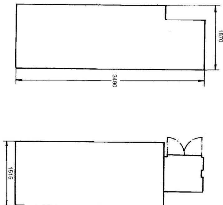
Рис.2 Габаритные размеры
