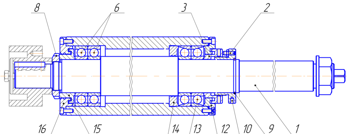
Рис. 27. Шпиндель
