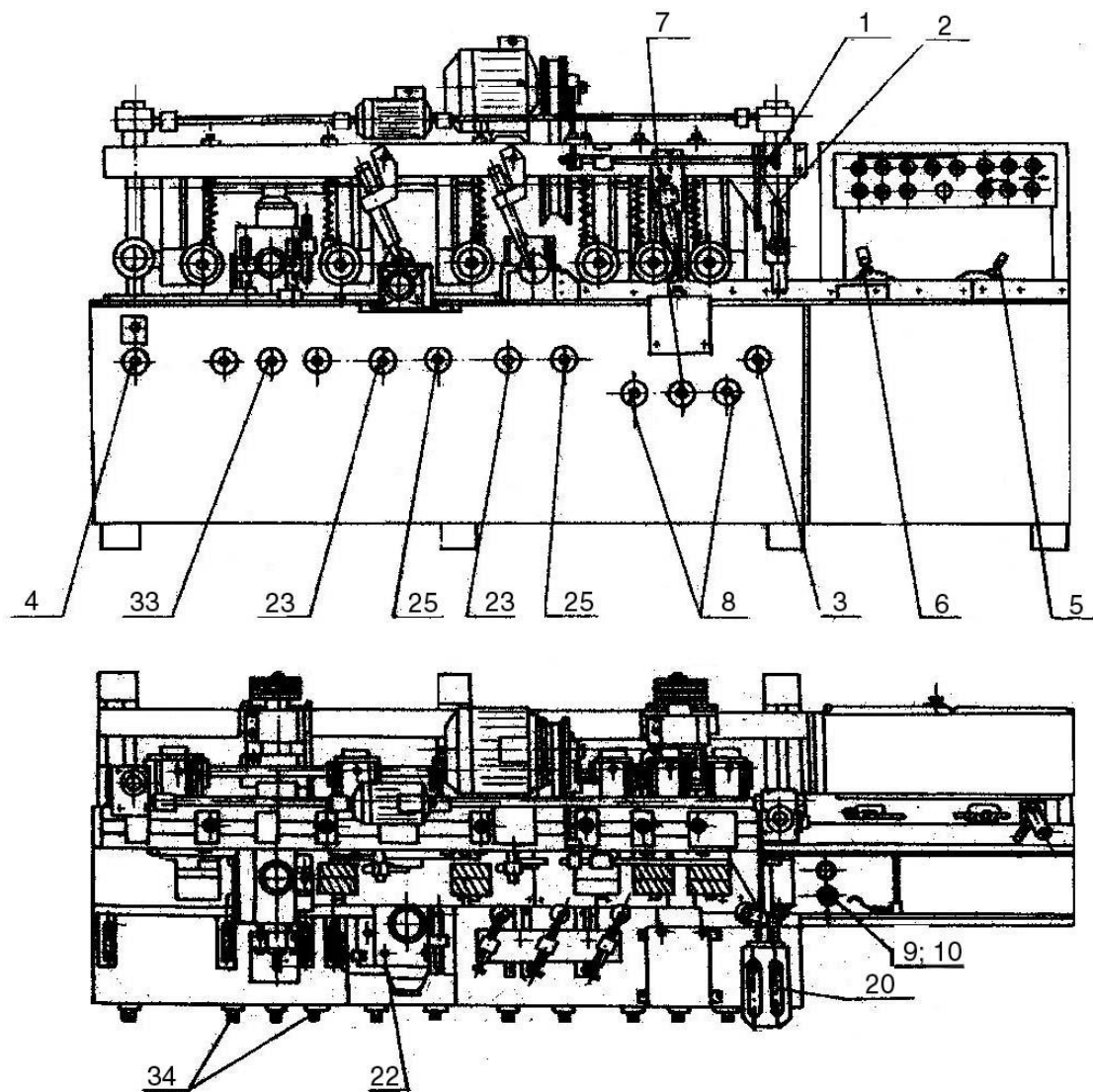
Рис.4 Расположение органов управления станка.
