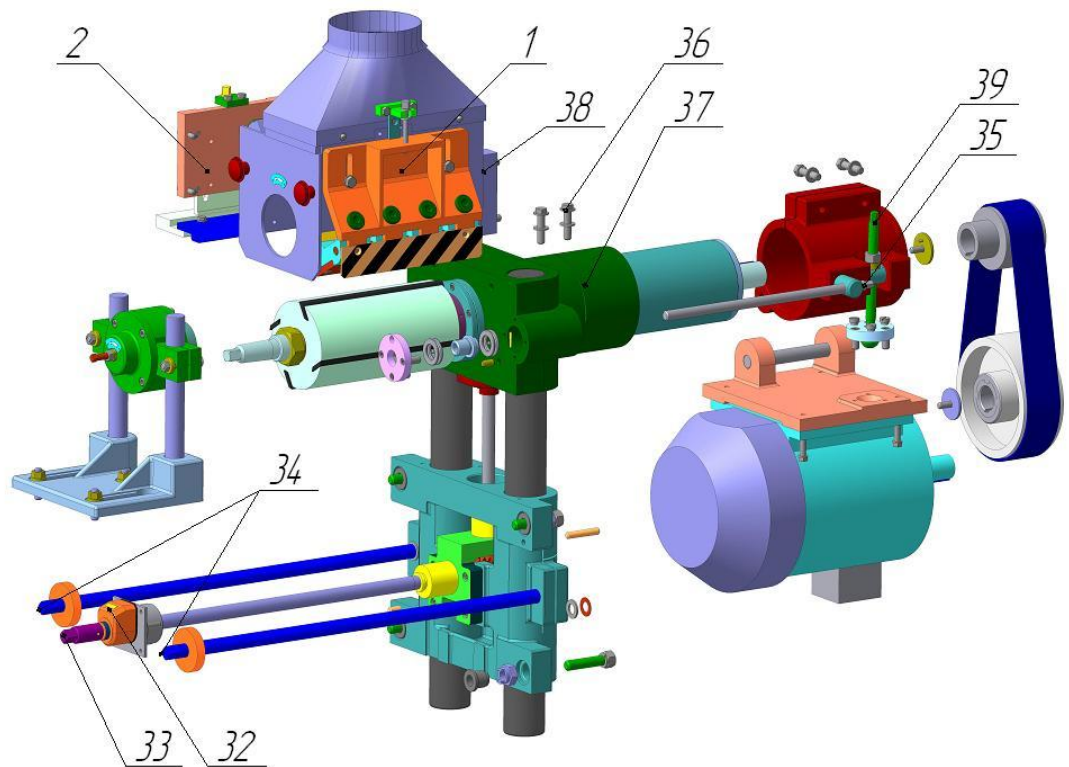
Рис. 15. Суппорт верхний
