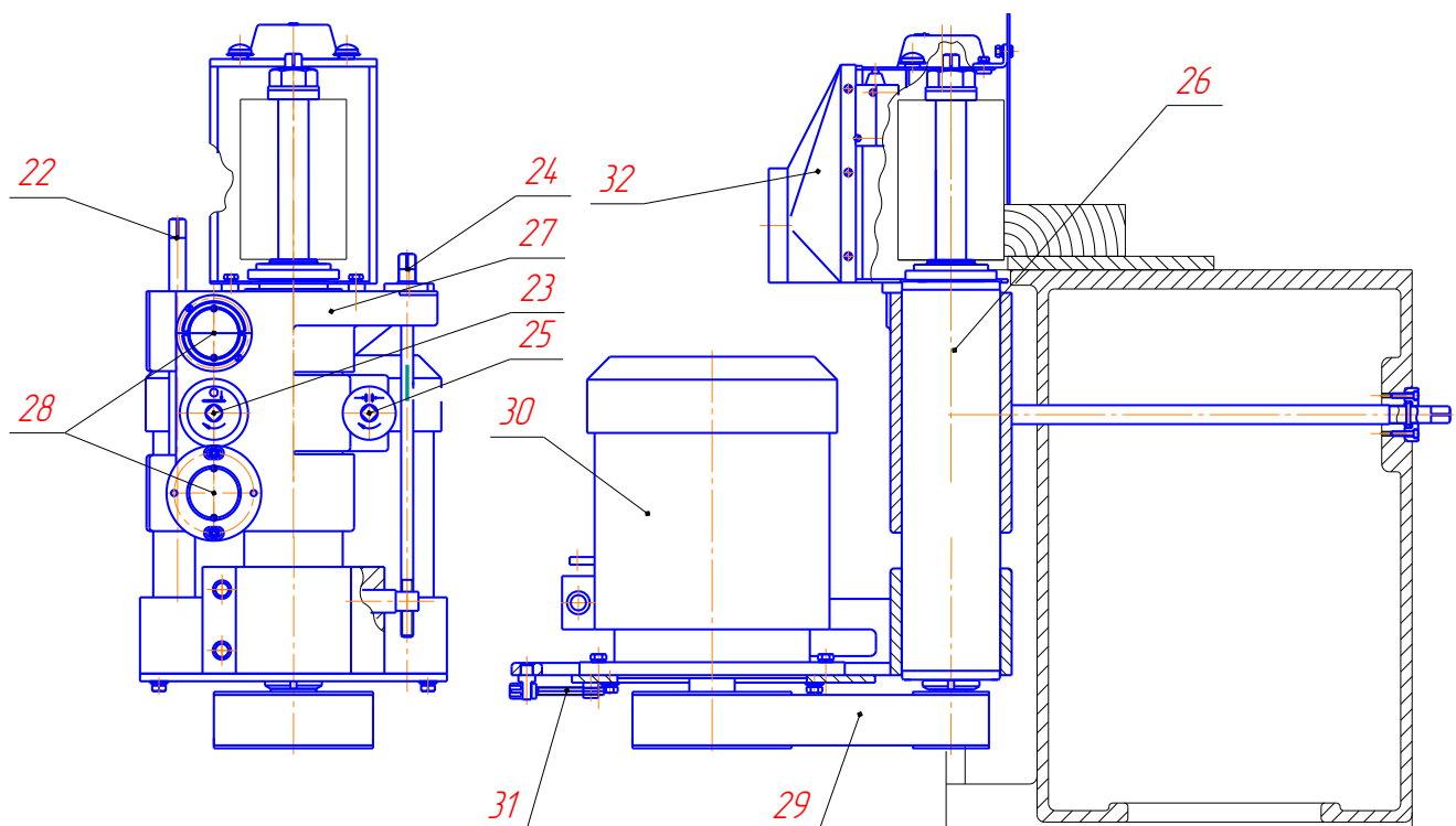
Рис. 13. Суппорт правый
