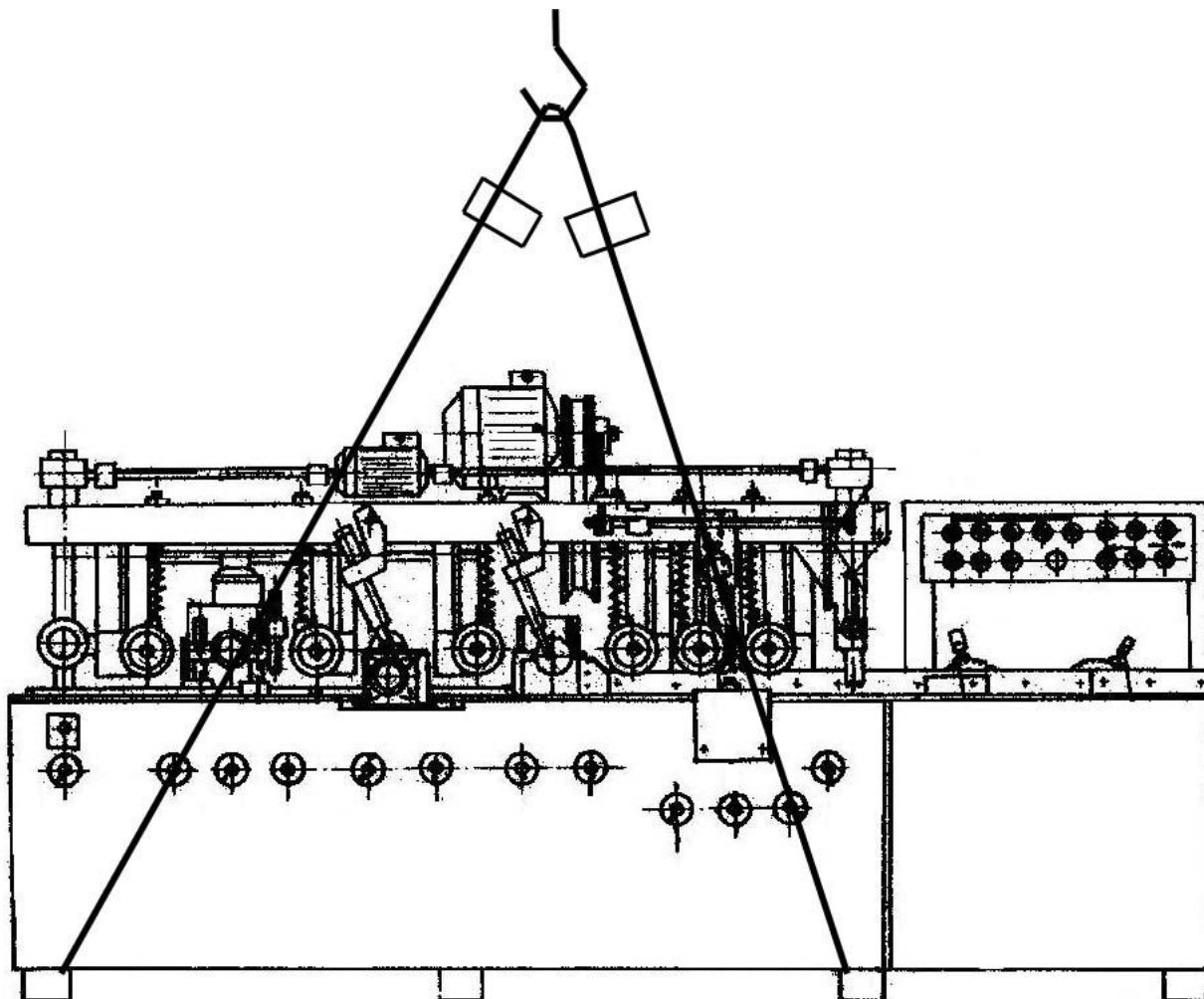
Рис. 23. Схема транспортировки станка
