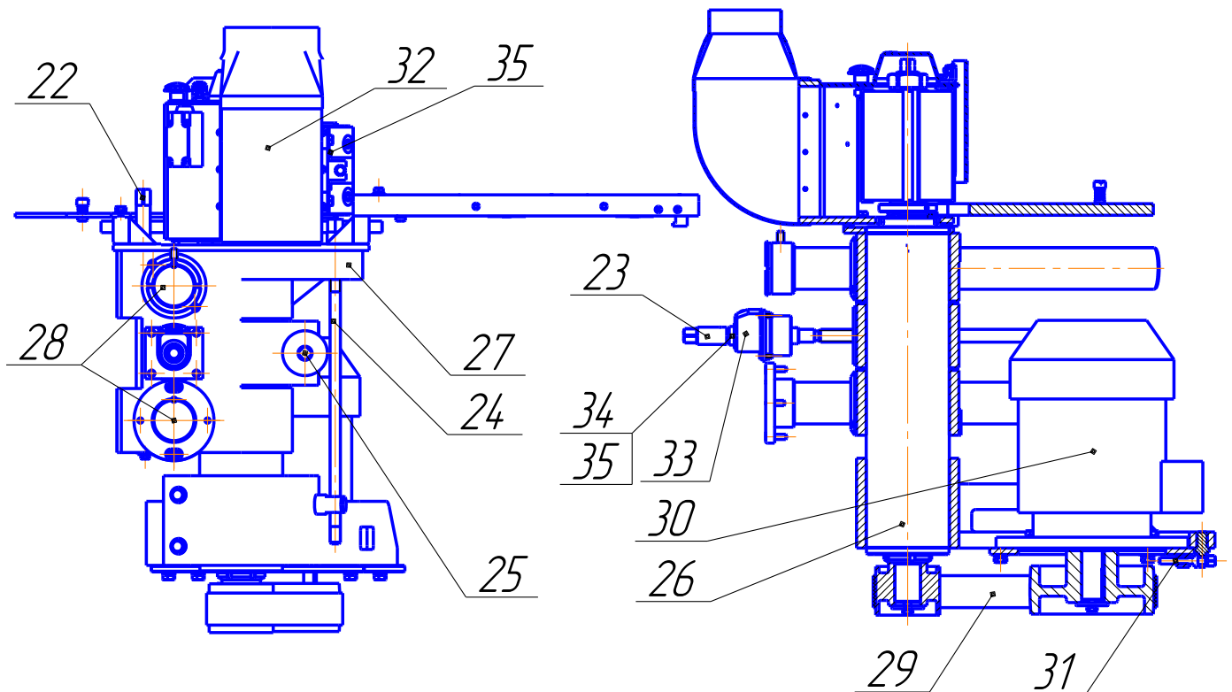
Рис. 14. Суппорт левый
