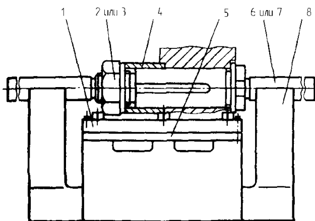
Рис. 4.5. Приспособление для установки ножей сборных фрез ИП.23.000
