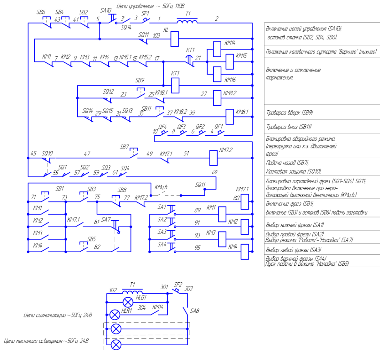
Рис. 19. Схема электрическая принципиальная станка модели C25-4M
