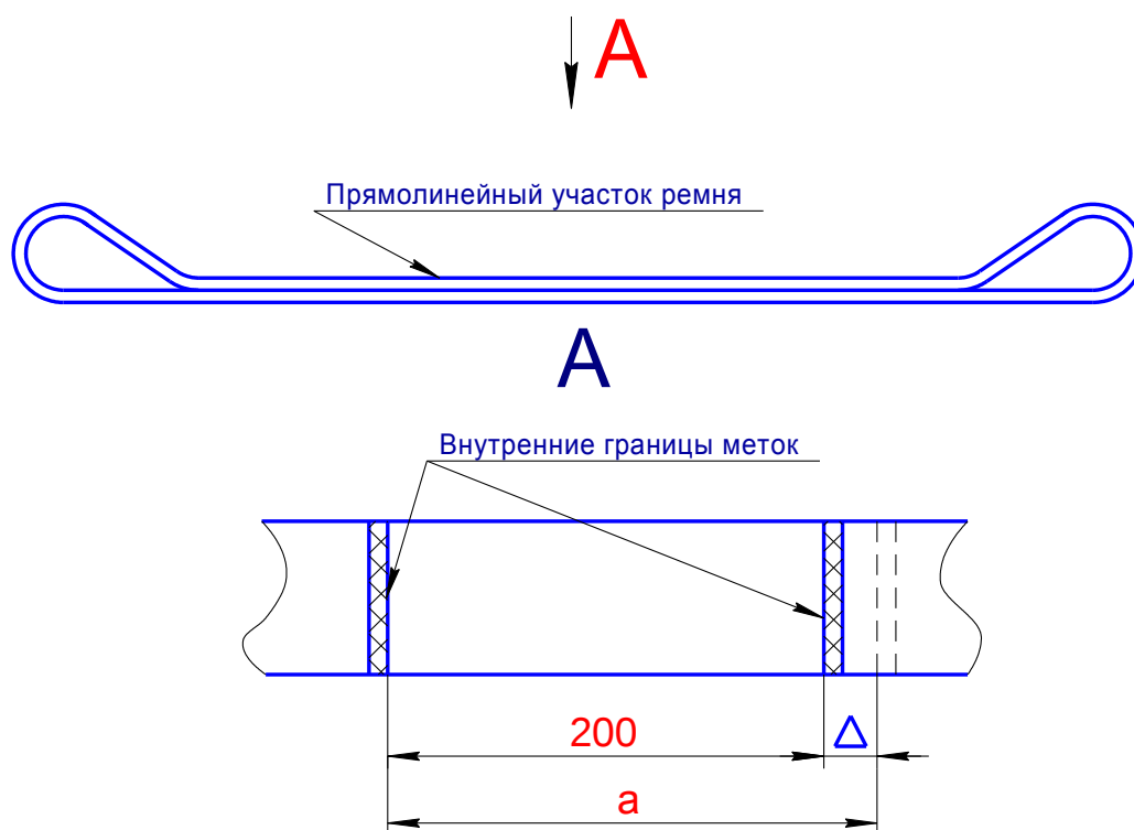
Рис. 28. Схема нанесения меток при натяжении нового ремня
