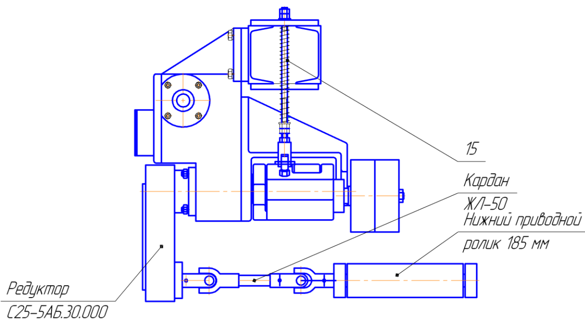
Рис. 9. Механизм подачи
