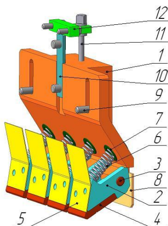
Рис. 16. Прижим передний
