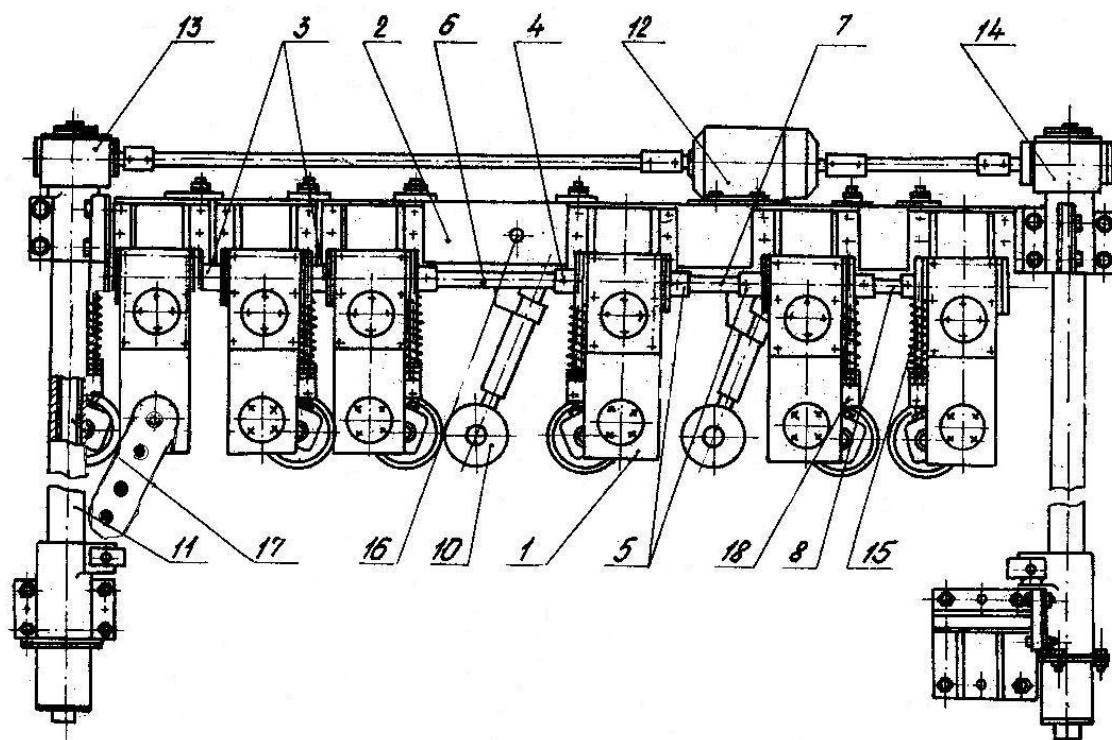
Рис. 8. Механизм подачи
