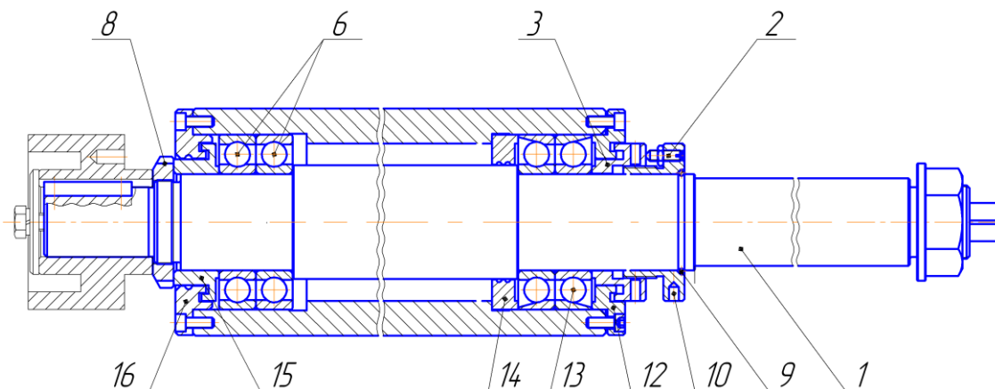
Рис. 27. Шпиндель
