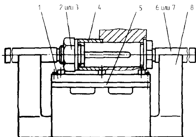
Рис. 4.5. Приспособление для установки ножей сборных фрез ИП.23.000
