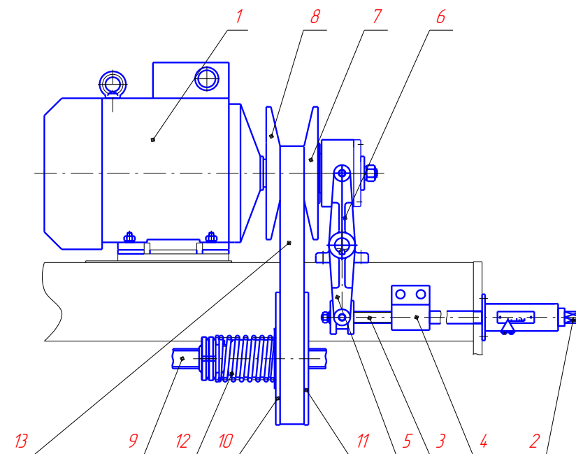
Рис. 7. Привод подачи
