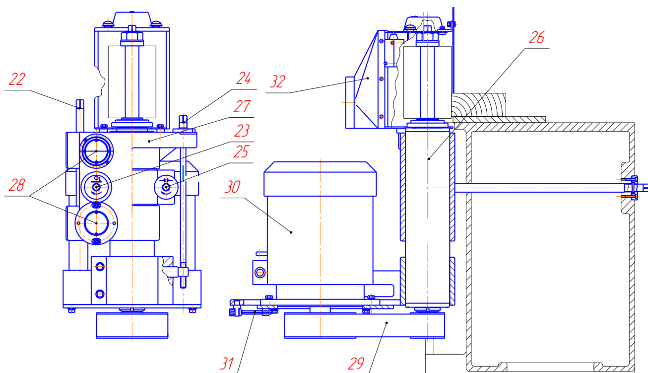
Рис. 13. Суппорт правый
