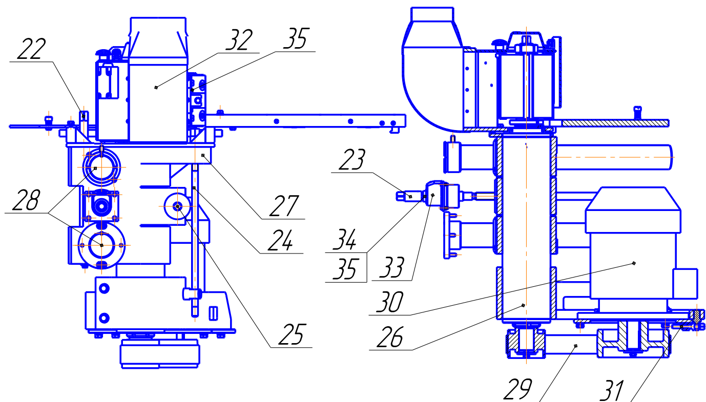
Рис. 14. Суппорт левый
