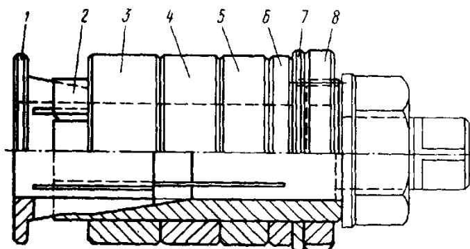
Рис. 4.1. Оправка ИП.01.000
