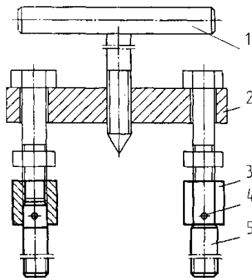
Рис. 4.4. Приспособление для снятия фрез ИП.12.000
