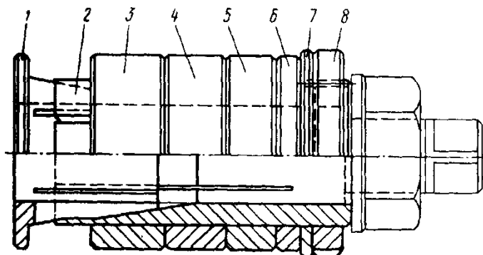
Рис. 4.2. Оправка цанговая правая ИП.07.000
