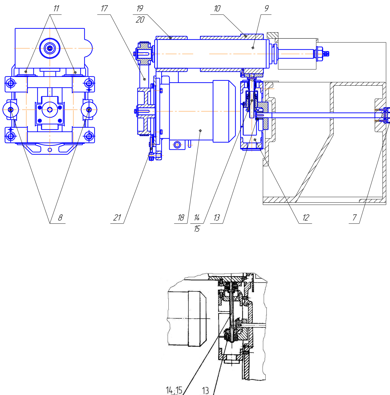
Рис. 12. Суппорт нижний
