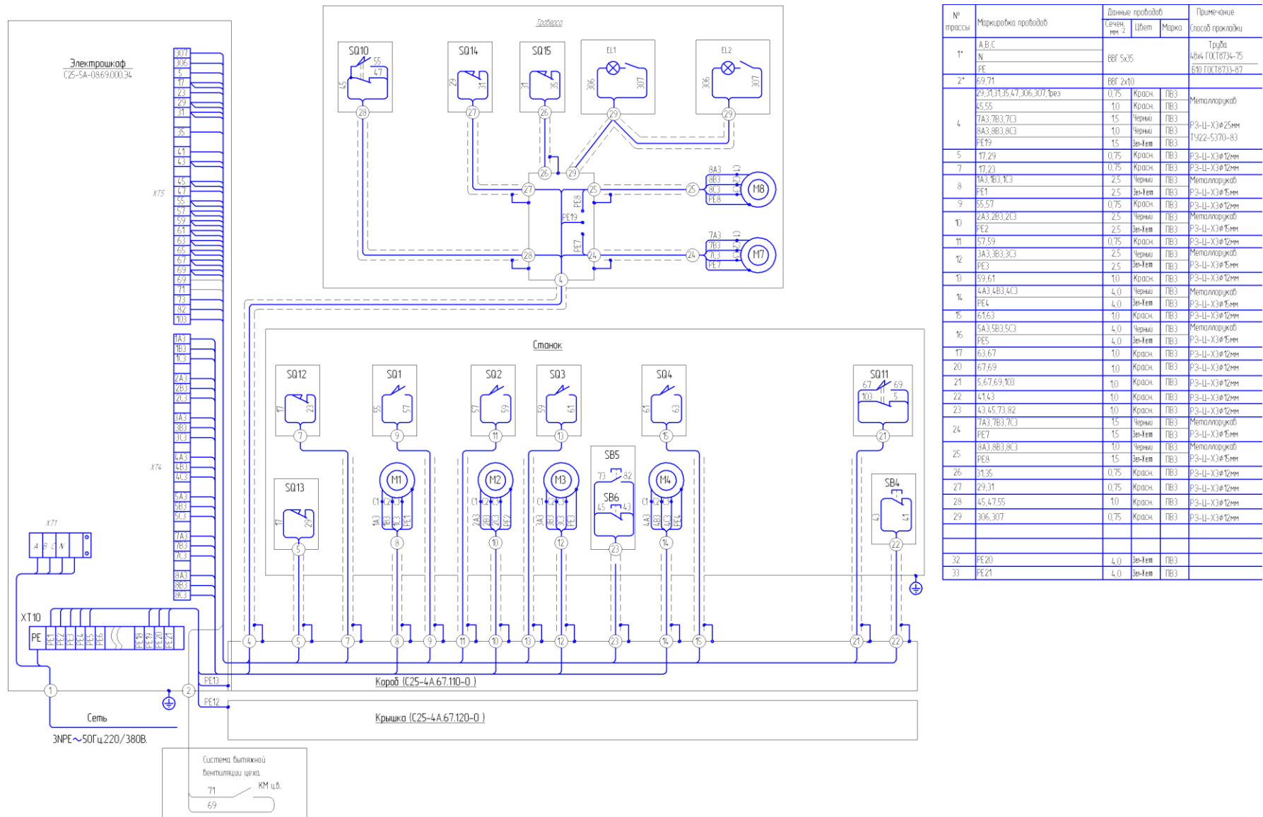
Рис. 20. Схема электрическая общая станка модели C25-4M
