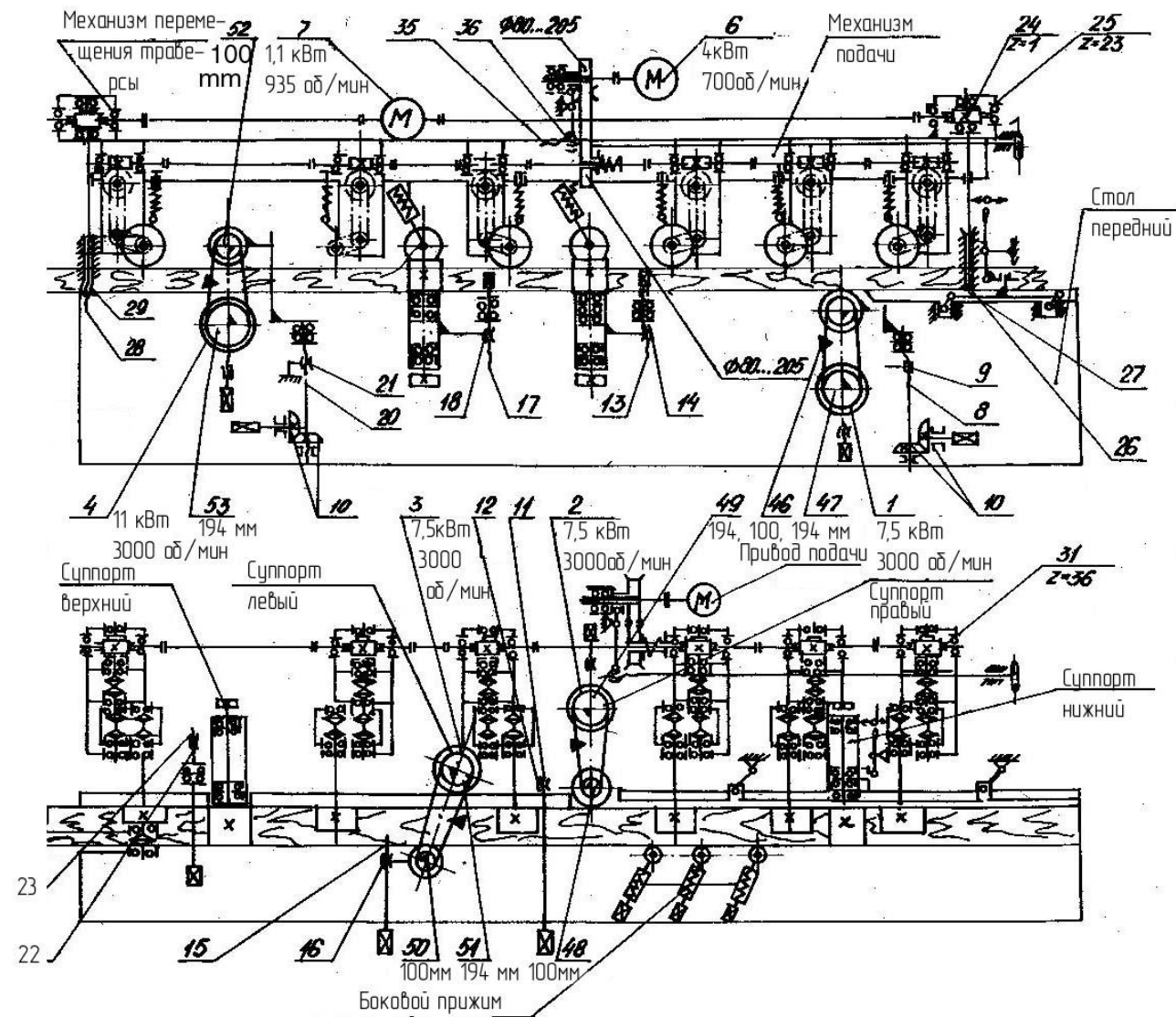
Рис. 6. Схема кинематическая станка С25-4М
